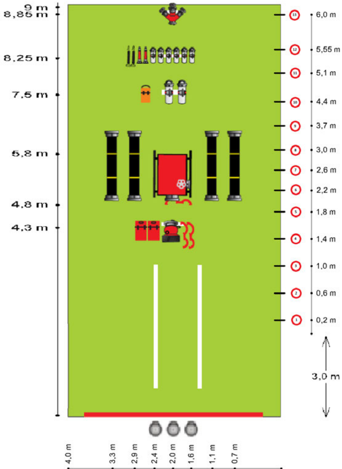
Slika 2: Pravilna postavitev orodja in opreme pri vaji Postavitev orodja za vajo z motorno brizgalno
