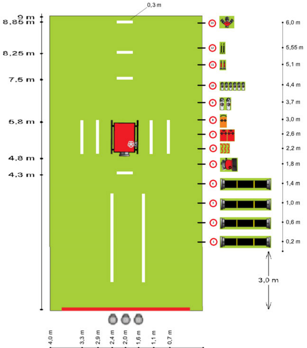
Slika 1: Tekmovalni prostor vaje Postavitev orodja za vajo z motorno brizgalno in začetna postavitev orodja, opreme ter tekmovalcev
